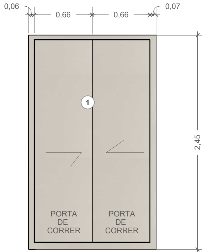
VISTA 01 ESC: 1:25
