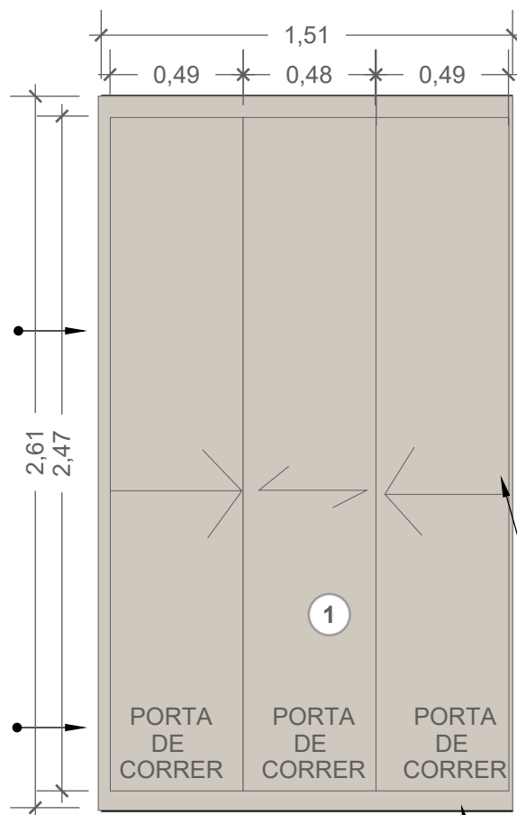
VISTA 01 ESC: 1:25
