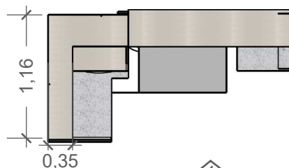
PLANTA ESC: 1:50
