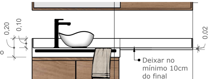
VISTA 01 ESC: 1:20
