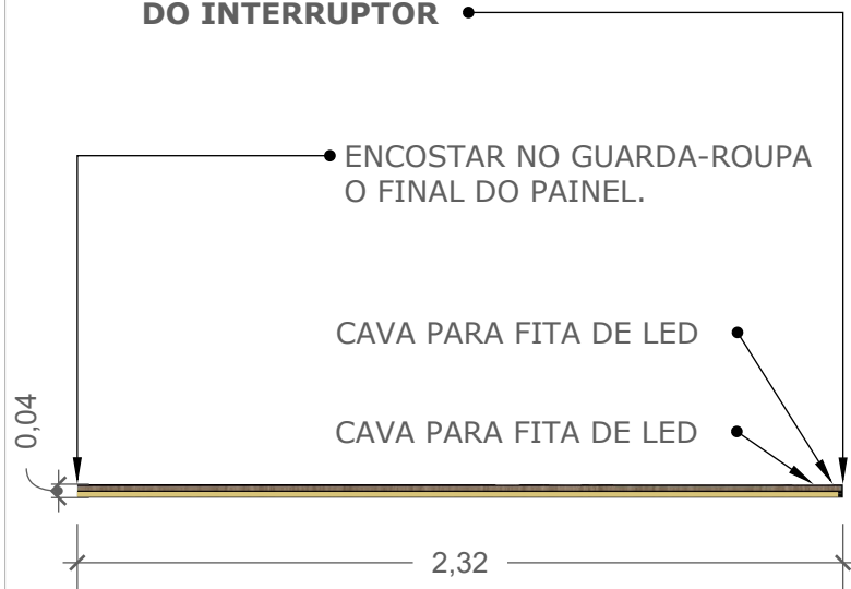
PLANTA ESC: 1:25
