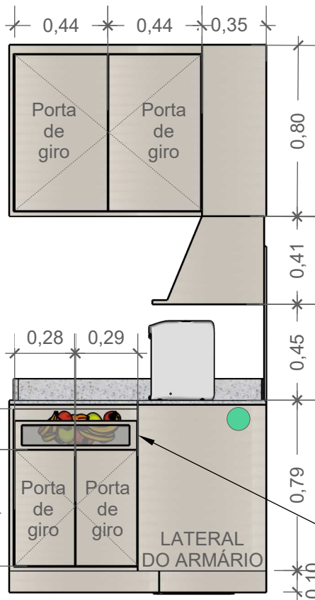
VISTA 01 ESC: 1:25
