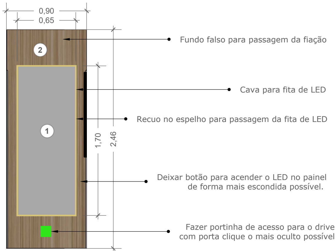
VISTA 01 ESC: 1:25
