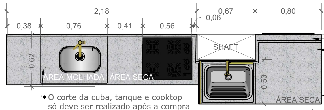
PLANTA - PIA COZINHA ESC: 1:25
