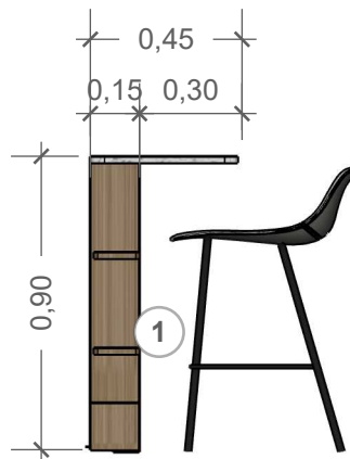
VISTA 03 ESC: 1:25
