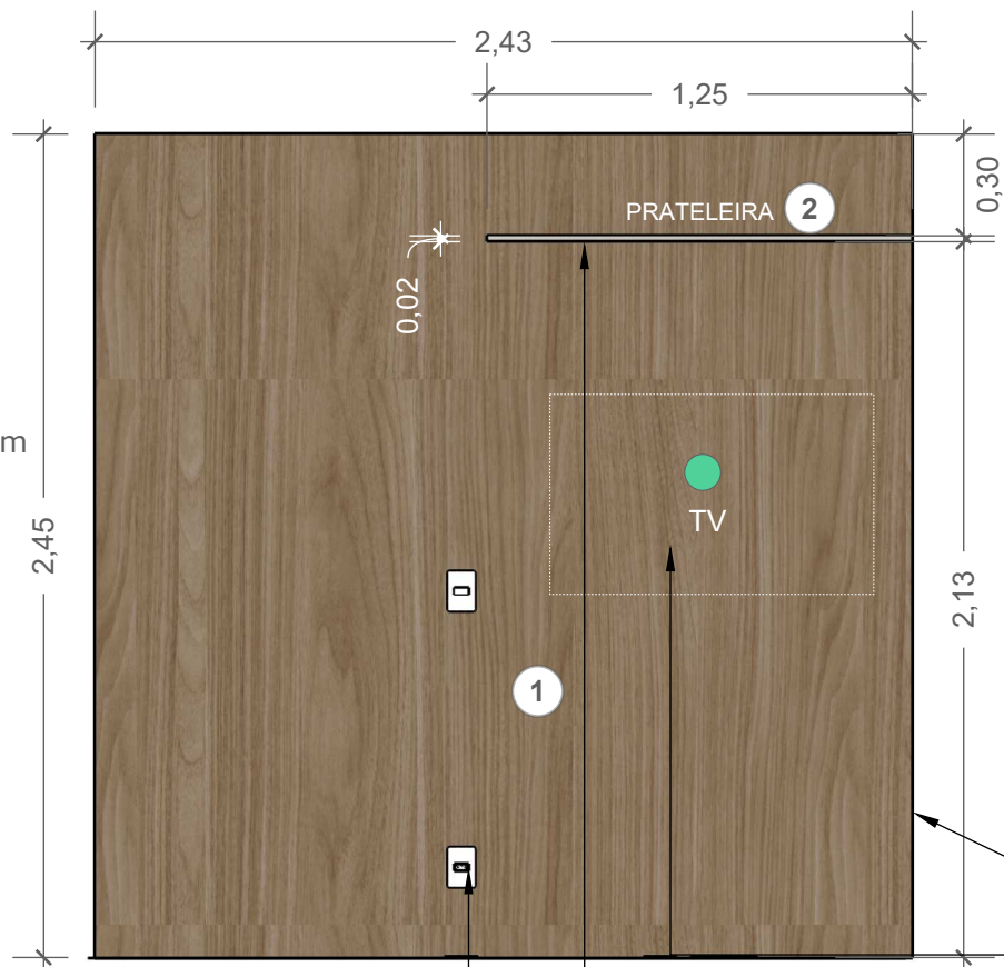
VISTA 01 ESC: 1:25
