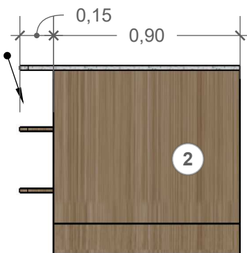
VISTA 01 ESC: 1:25
