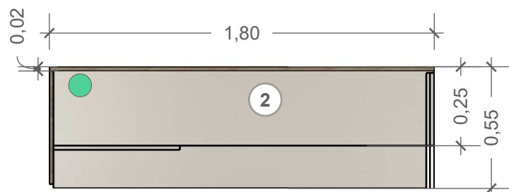
PLANTA ESC: 1:25
