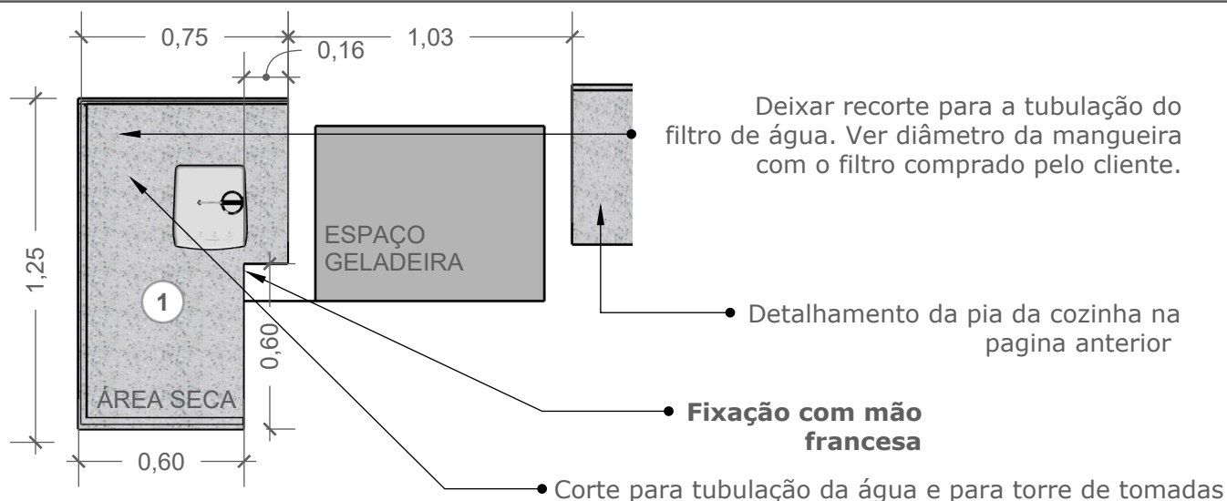
PLANTA - EXTENSÃO DA PIA DA COZINHA ESC: 1:25
