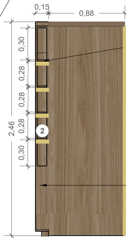
VISTA 02 ESC: 1:25
