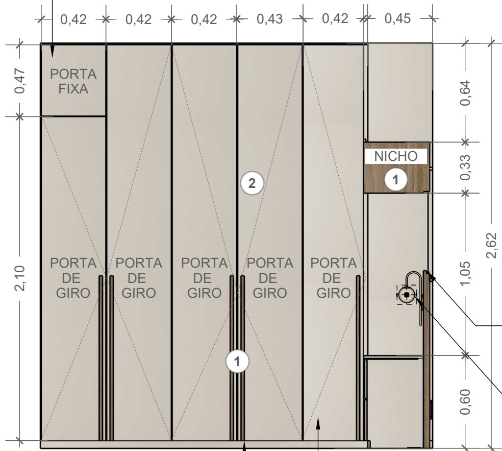
VISTA 02 ESC: 1:25
