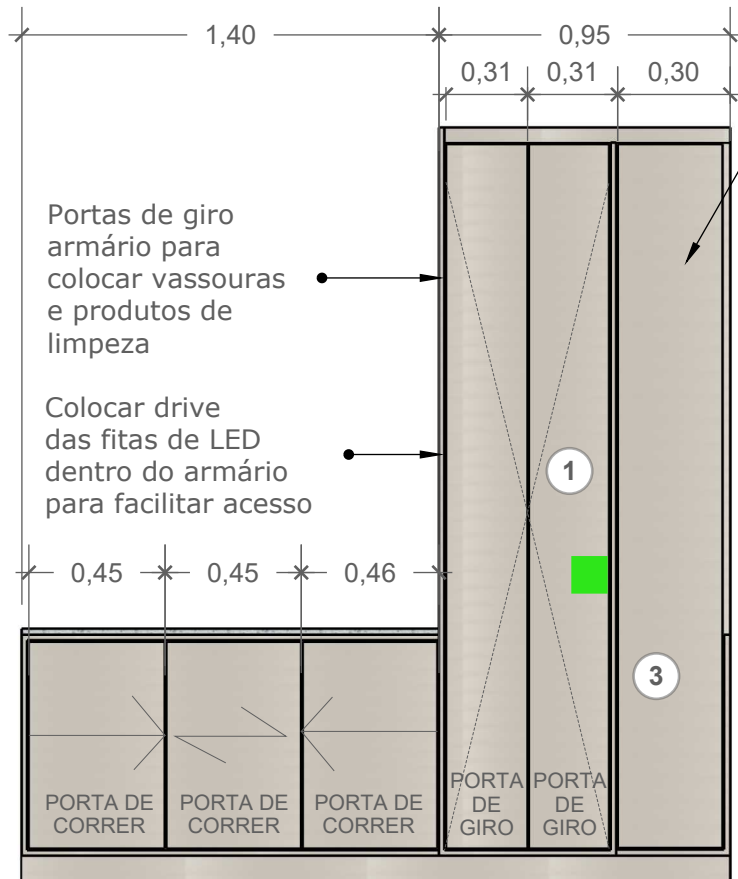
VISTA 01 ESC: 1:25
