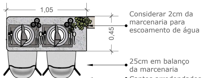
PLANTA - ARMÁRIO DA FRENTE DA PIA DA COZINHA ESC: 1:25
